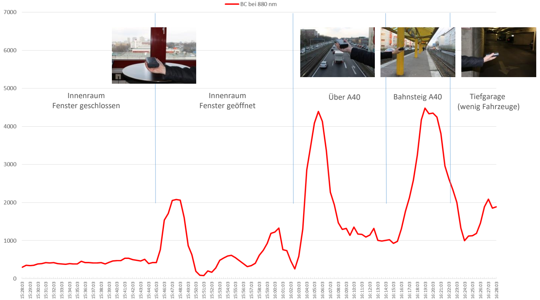
Mobile Messungen mit einem MA200 im und am ETEC; Datum: 30.01.2018 in [ng/m 3 ]:
